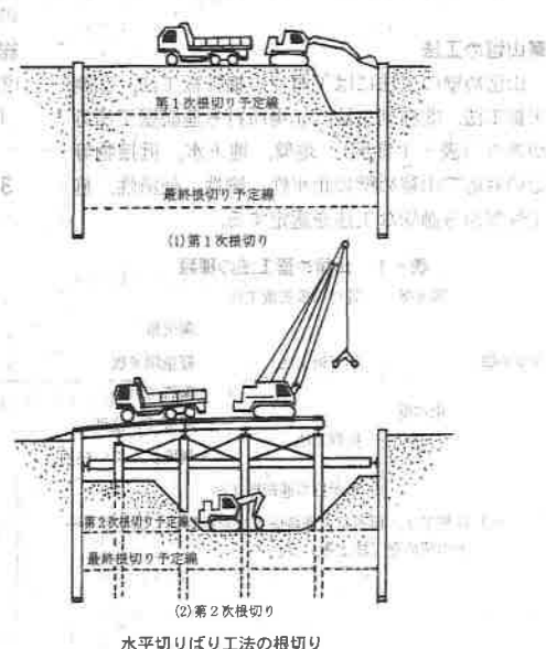
(2)第2次根切り 水平切りばり工法の根切り
